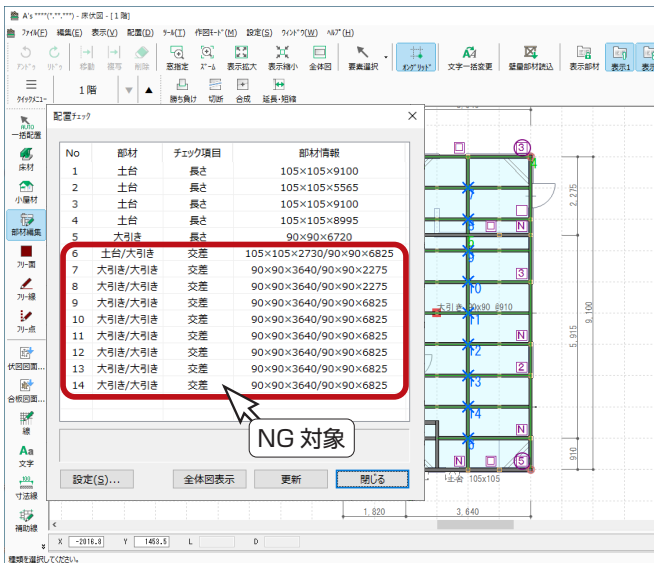
1 階床伏図
